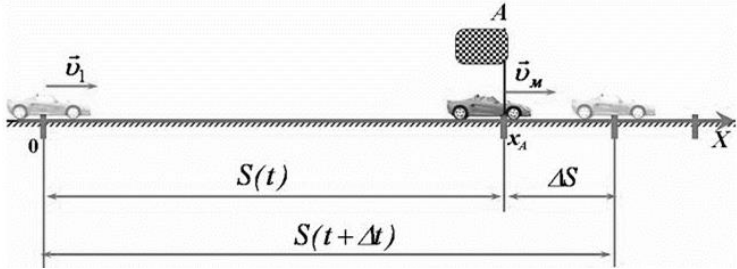
Рис. 1. Рух автомобіля
