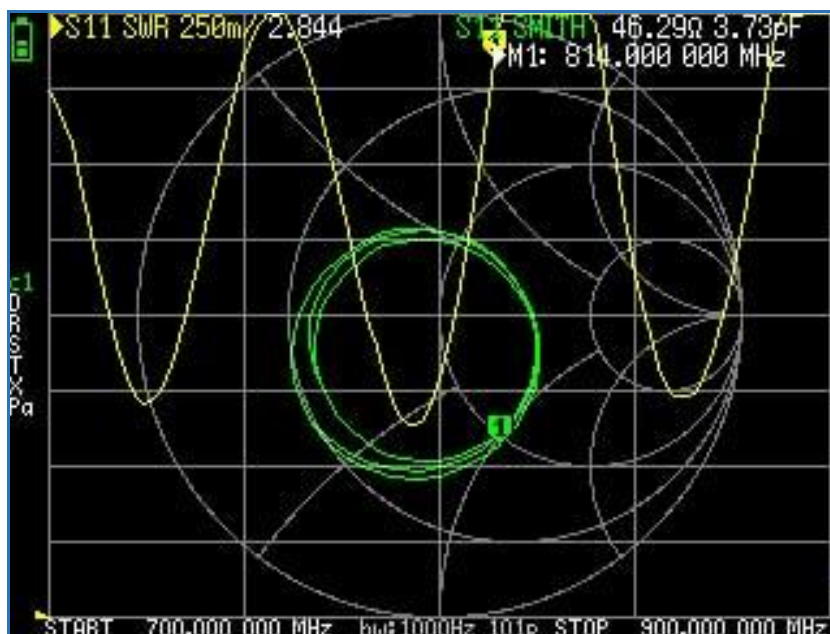
Рис. 2. Характеристика антени Фібоначі
